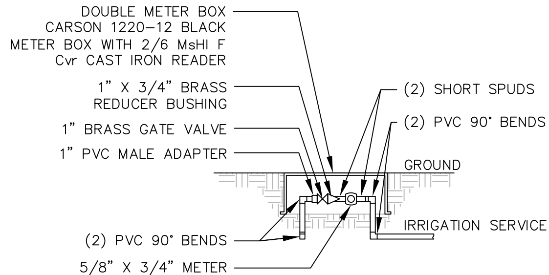
SECTION A-A
